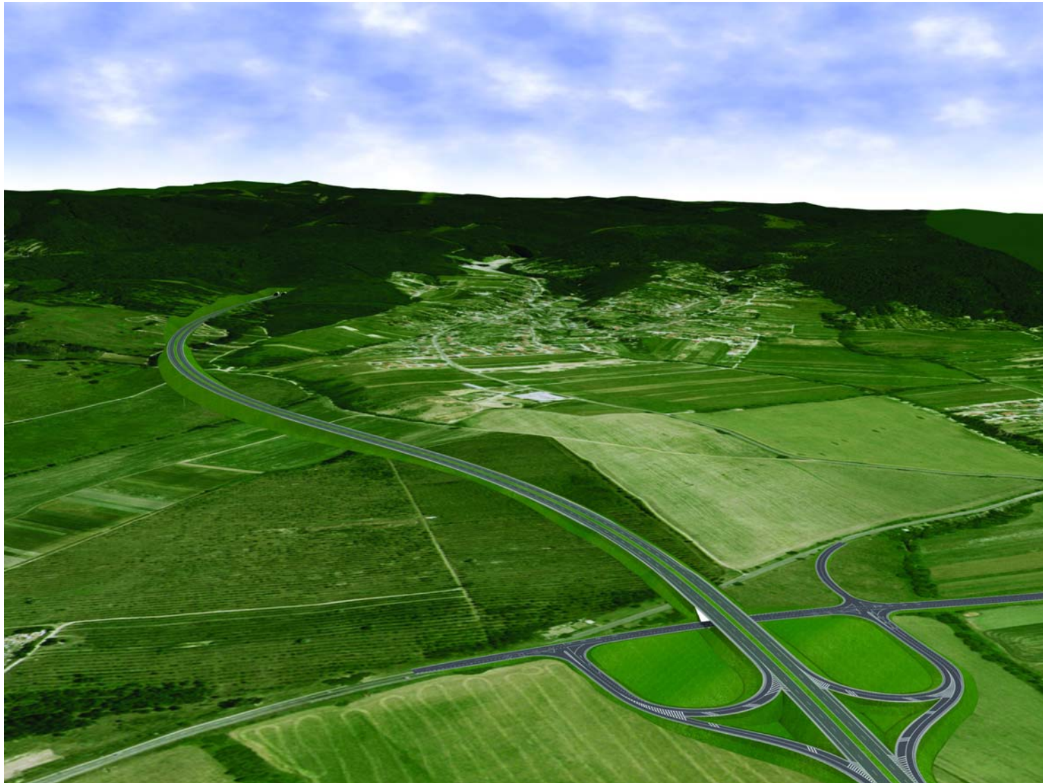
Obr. 4: Variant 2 – MÚK Záhorská Bystrica a pohľad na Marianku
