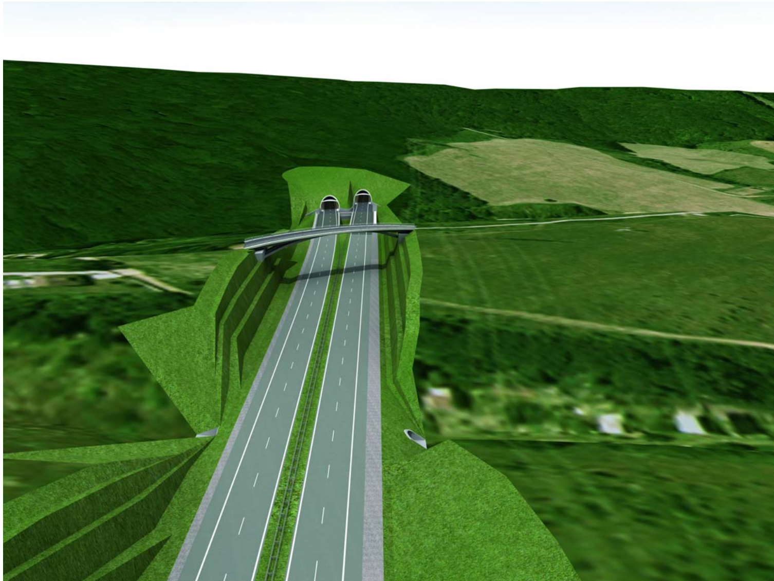
Obr. 10: Variant 3 – portál druhého tunela u Borinky
