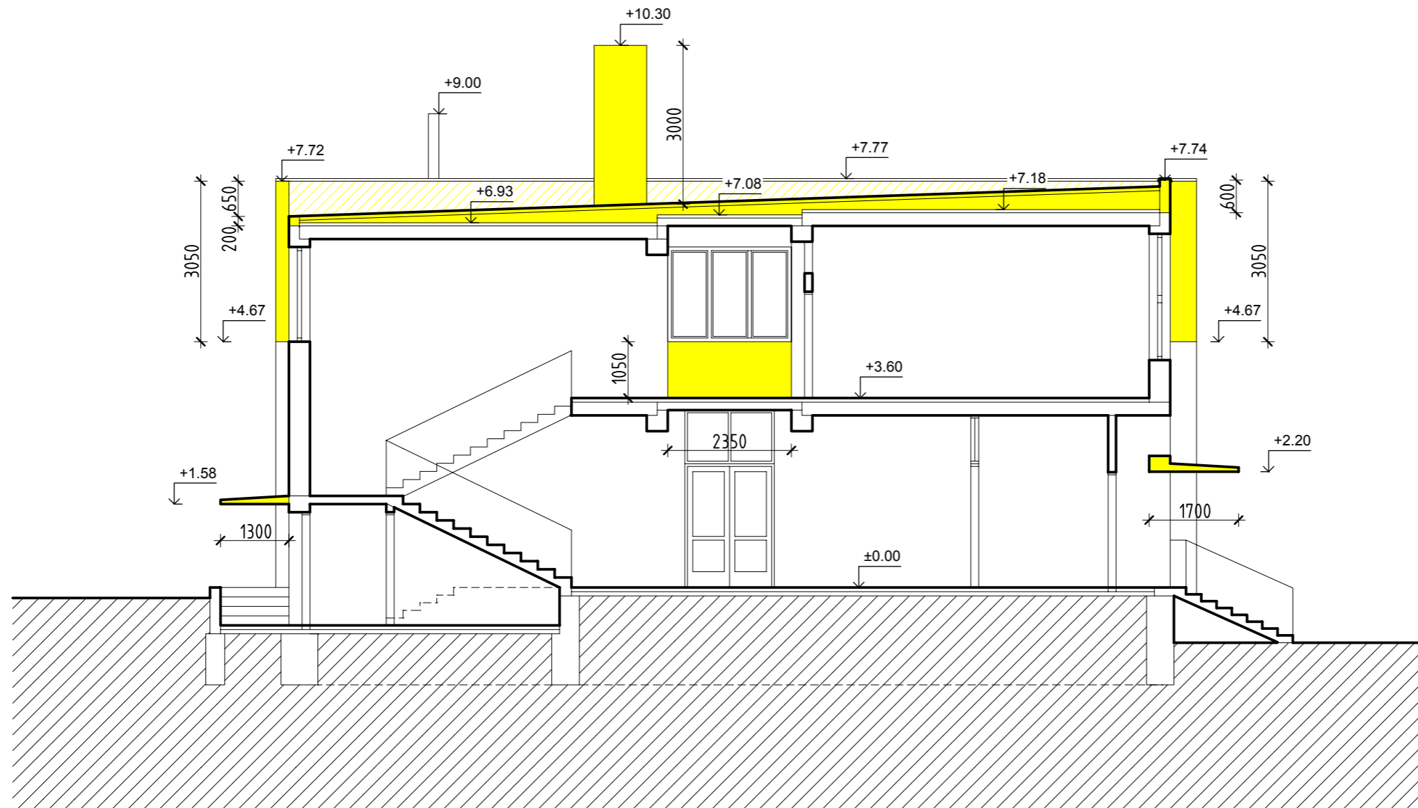
REZ B-B
