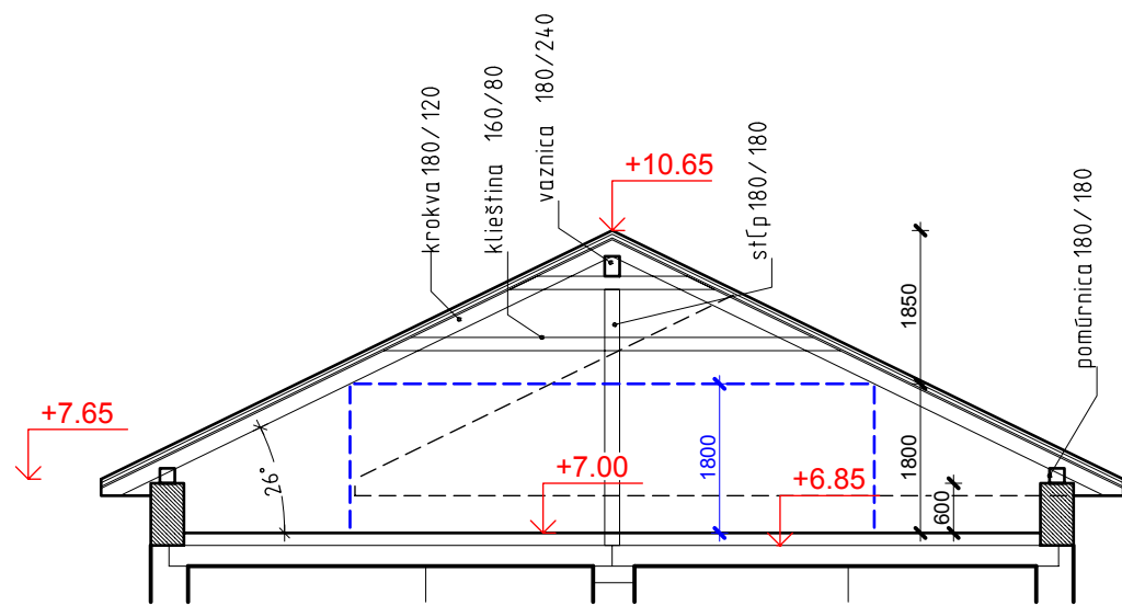
Rez B-B
