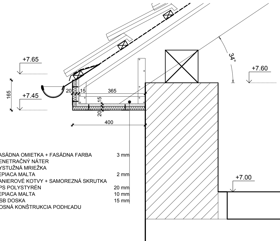
DETAIL D1 V MIESTE OKAPU M 1:10
